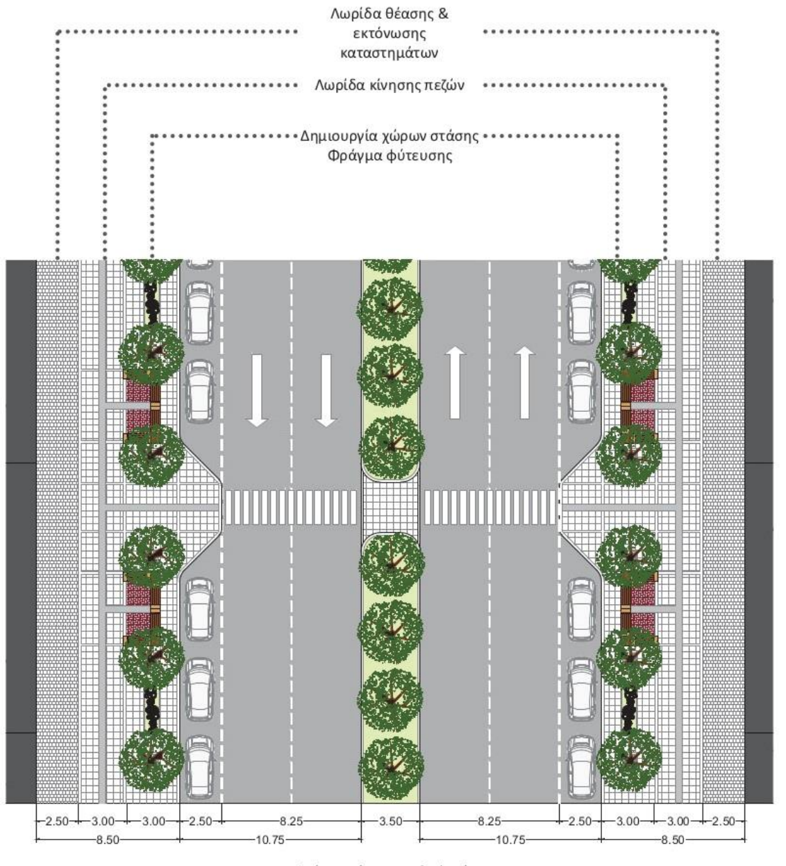
ΕΝΔΕΙΚΤΙΚΗ ΔΙΑΜΟΡΦΩΣΗ ΤΜΗΜΑΤΟΣ ΛΕΩΦΟΡΟΥ ΒΕΪΚΟΥ
